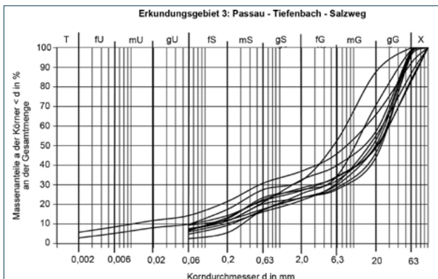
Abb. 7-18: Kornverteilung der untersuchten Kiese der Bohrungen Q 28, Q 29, Q 30 u. Q 31 sowie der Kiesgruben Nr. 24 Salzweg W und Nr. 29 Schmidöd.
