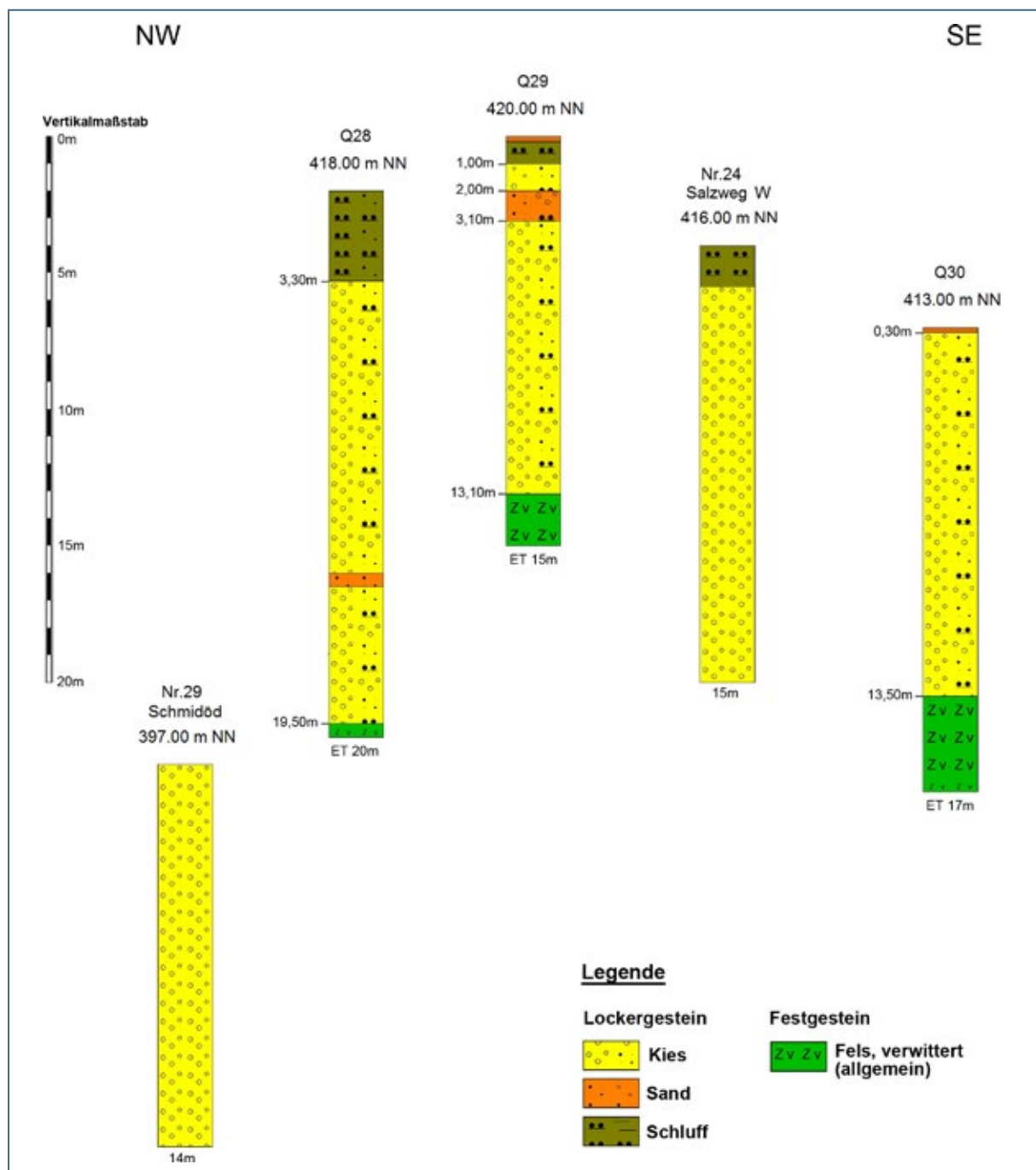
Abb. 7-17: Profilschnitt im Bereich östlich der Ilz bzw. nördlich Passau im Erkundungsgebiet 3. Kieshorizonte mit Meterangabe unter Ansatzpunkt; mNN = Meter über Normal Null, ET = Endteufe
