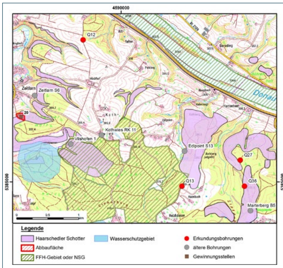
Abb. 7-9: Lage der Erkundungsbohrungen Q 12, Q 13, Q 27, Q 36, vier älterer Forschungsbohrungen sowie der Gewinnungsstelle Nr. 20 Zeitlarn S.
