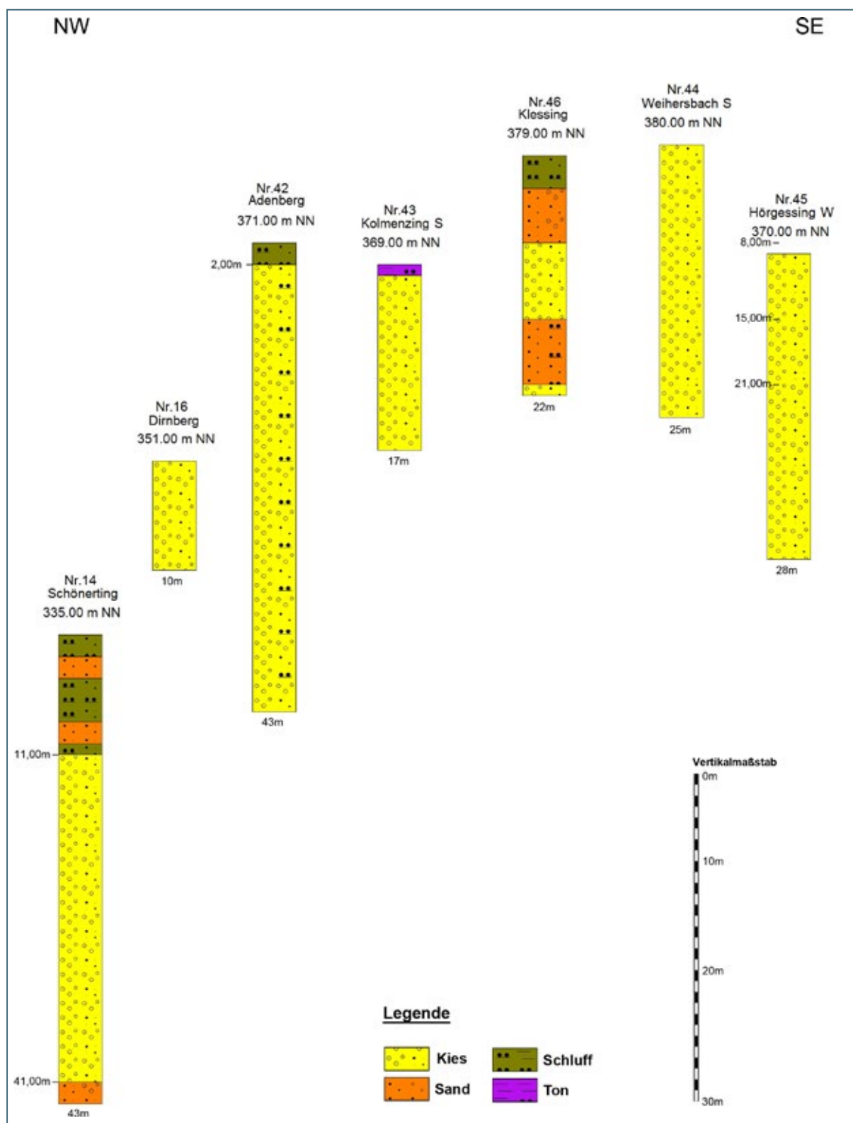
Abb. 7-43: Profilschnitt durch mehrere Kies- und Sandgruben zwischen nördlich und südlich der Vils . mNN = Meter über Normal Null
