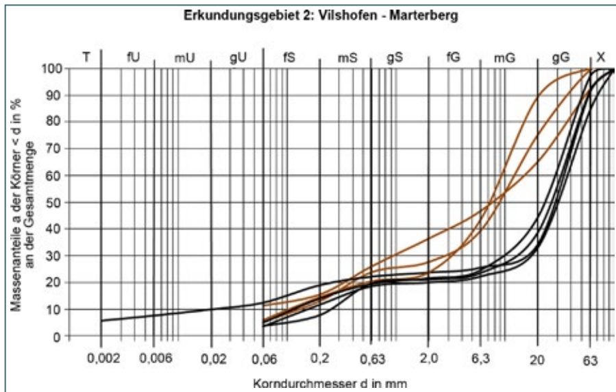
Abb. 7-11: Kornverteilung der untersuchten Kiesproben aus den Bohrungen Q 12, Q 13, Q 27, Q 36. Schwarze Kurven repräsentieren Grobkiese, braune Summenkurven Fein- bis Mittelkiese
