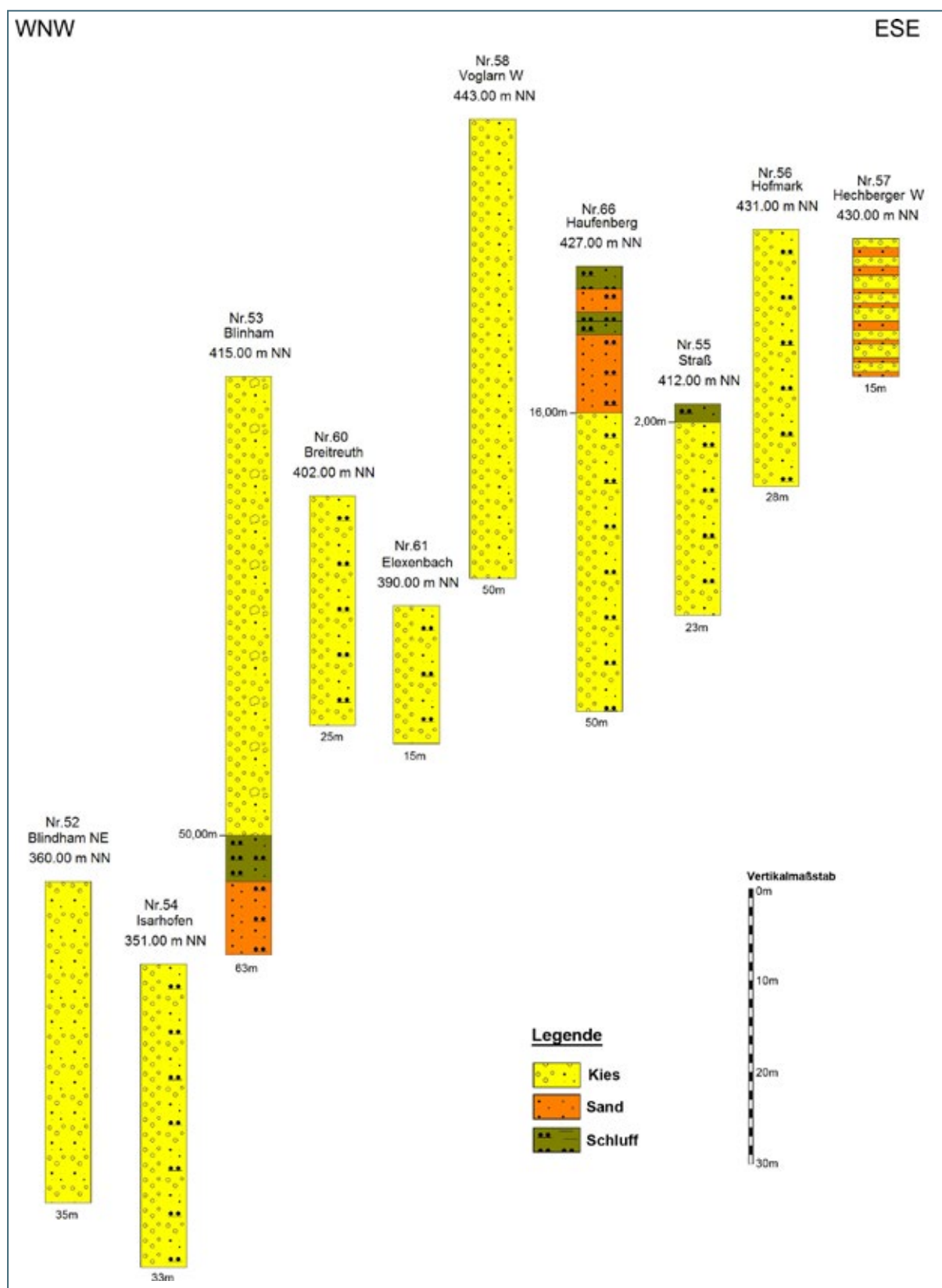
Abb. 7-45: Profilschnitt durch mehrere Kies- und Sandgruben östlich von Ortenburg. mNN = Meter über Normal Null
