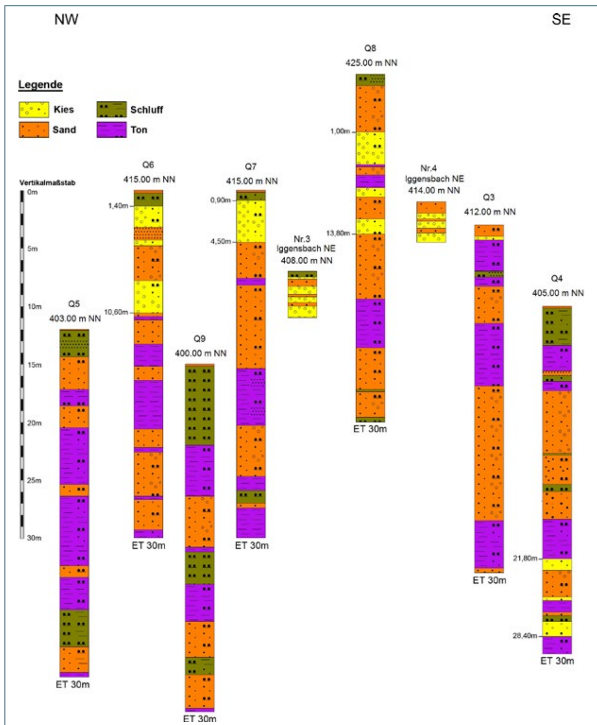
Abb. 7-5: Profilschnitt im Bereich Iggensbach - Schöllnach. Kiesbereiche mit Meterangabe unter Ansatzpunkt; mNN = Meter über Normal Null, ET = Endteufe
