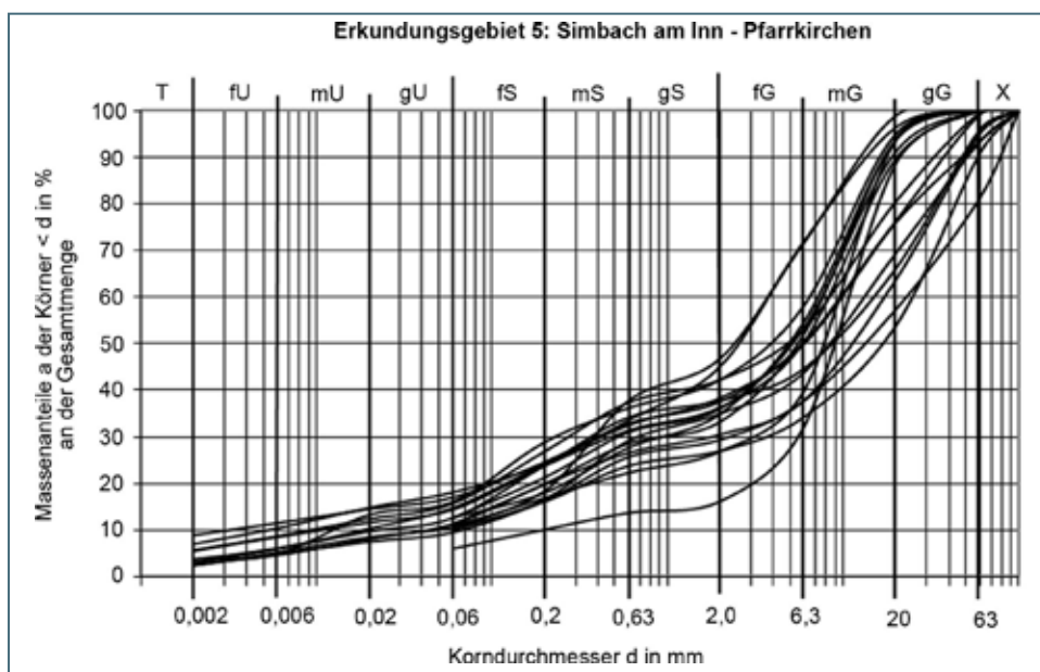
Abb. 7-32: Kornverteilung der untersuchten Kiese der Bohrungen Q 22, Q 23, Q 24, Q 25, Q 26, Q 34 und Q 35 sowie der Kiesgrube Nr. 107 Griesingsreith (Kößlarn) im Erkundungsgebiet 5.
