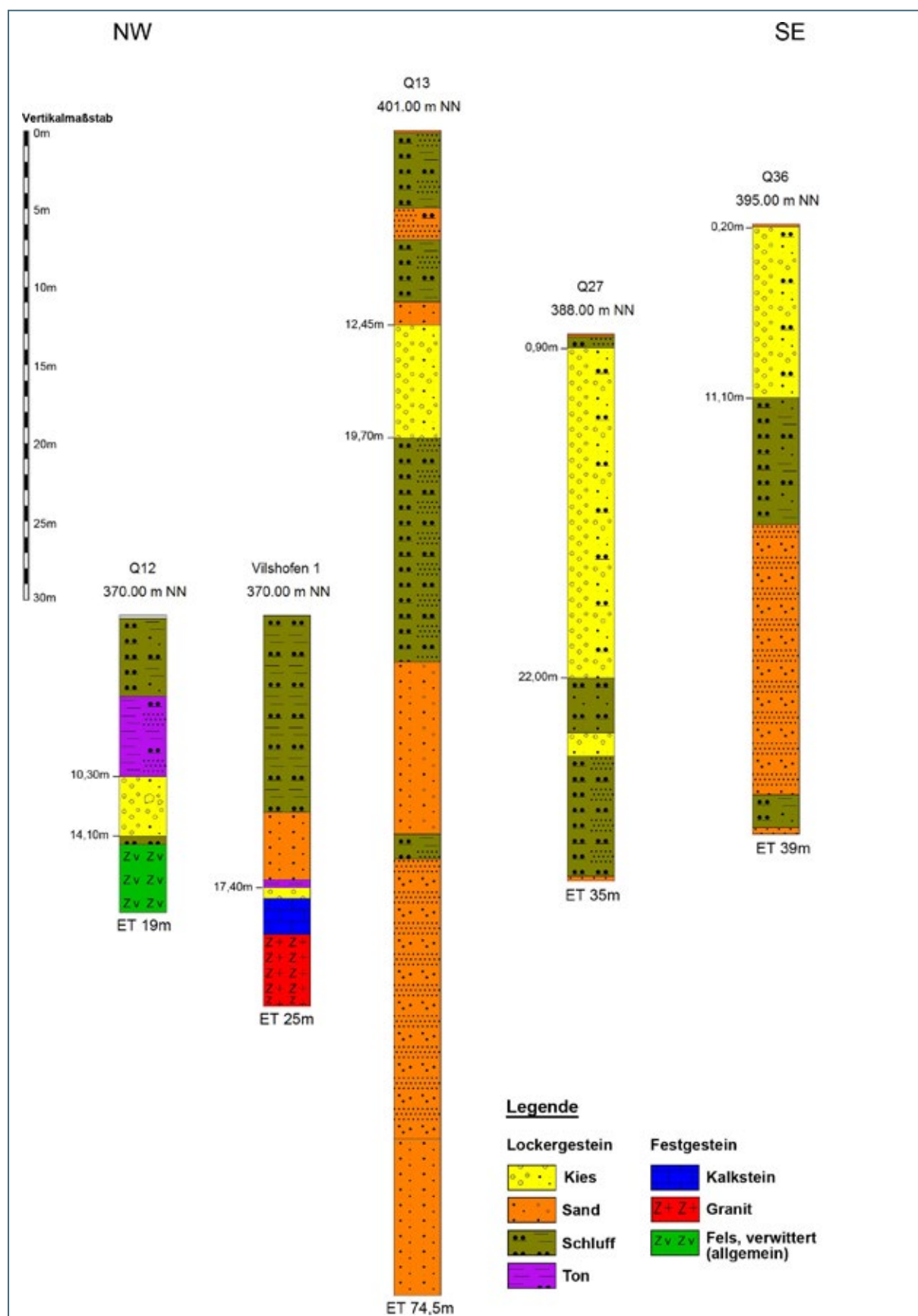
Abb. 7-10: Profilschnitt südlich der Donau mit einer Forschungsbohrung und den Erkundungsbohrungen. Kies-horizonte mit Meterangabe unter Ansatzpunkt; mNN = Meter über Normal Null, ET = Endteufe
