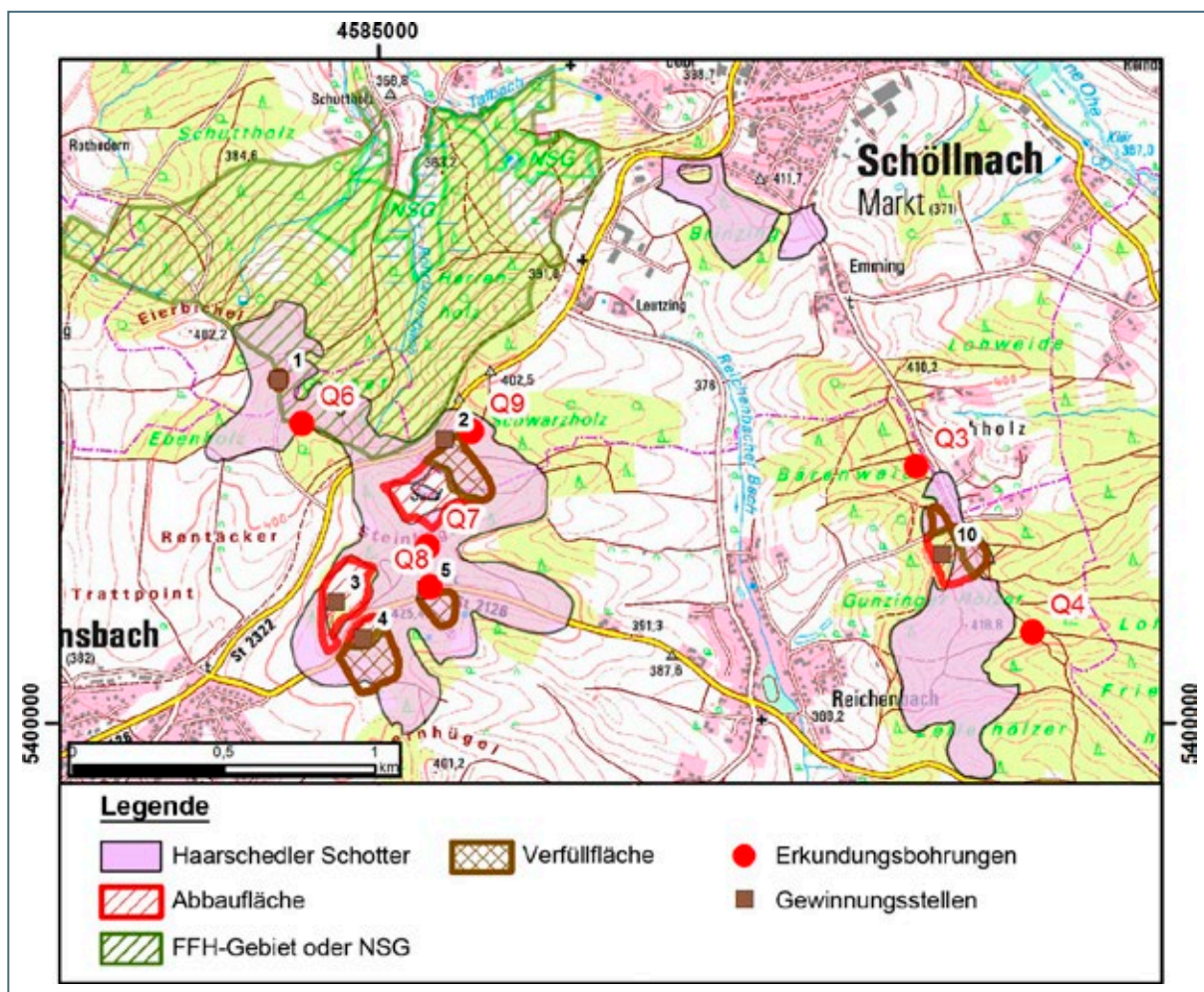
Abb. 7-4: Lage der Bohrungen (Q 3, Q 4, Q 6, Q 7, Q 8, Q 9) und Gewinnungsstellen (Nr. 1 – 5 und Nr. 10) bei Schöllnach.
