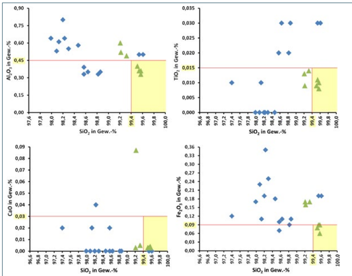
Abb. 7-41: Zusammenfassende Darstellung der chemischen Untersuchungsergebnisse aller Vollanalysen (blaue Rauten) und halbquantitativen Analysen (grüne Dreiecke) im Erkundungsgebiet 6
