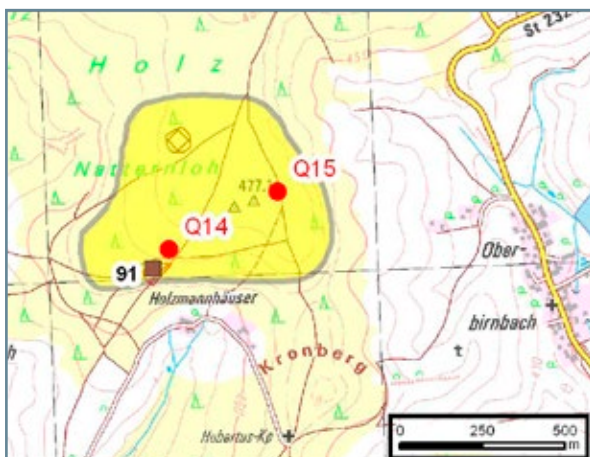
Abb. 8-5: Rohstoffpotenzialfläche Tattenbacher Holz
