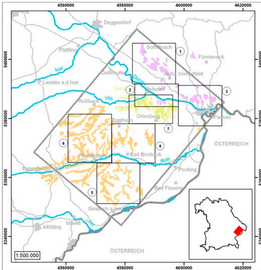
Abb. 3-1: Übersichtslageplan mit Lage der Erkundungsgebiete auf Quarzkiesvorkommen (rosa = Haarschedler Schotter, orange = Quarzrestschotter, gelbgrün = Ortenburger Schotter)
