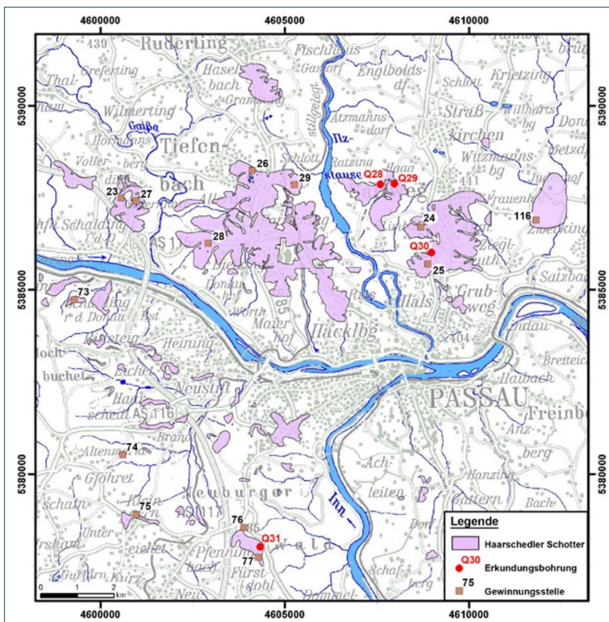
Abb. 7-14: Erkundungsgebiet 3: Passau – Tiefenbach – Salzweg.
