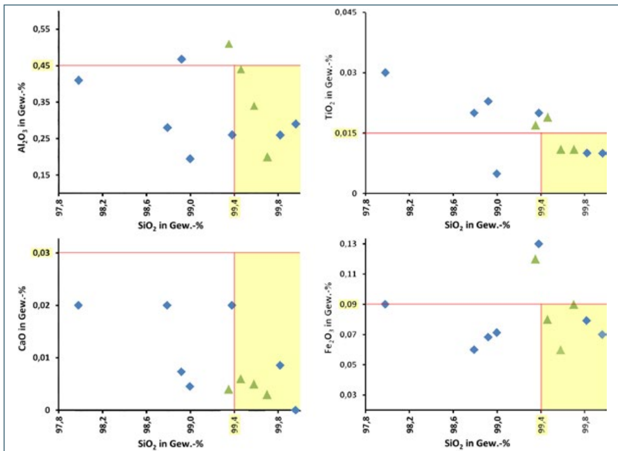
Abb. 7-7: Zusammenfassende Darstellung der chemischen Untersuchungsergebnisse aller Vollanalysen (blaue Rauten) und halbquantitativen Analysen (grüne Dreiecke) im Erkundungsgebiet 1
