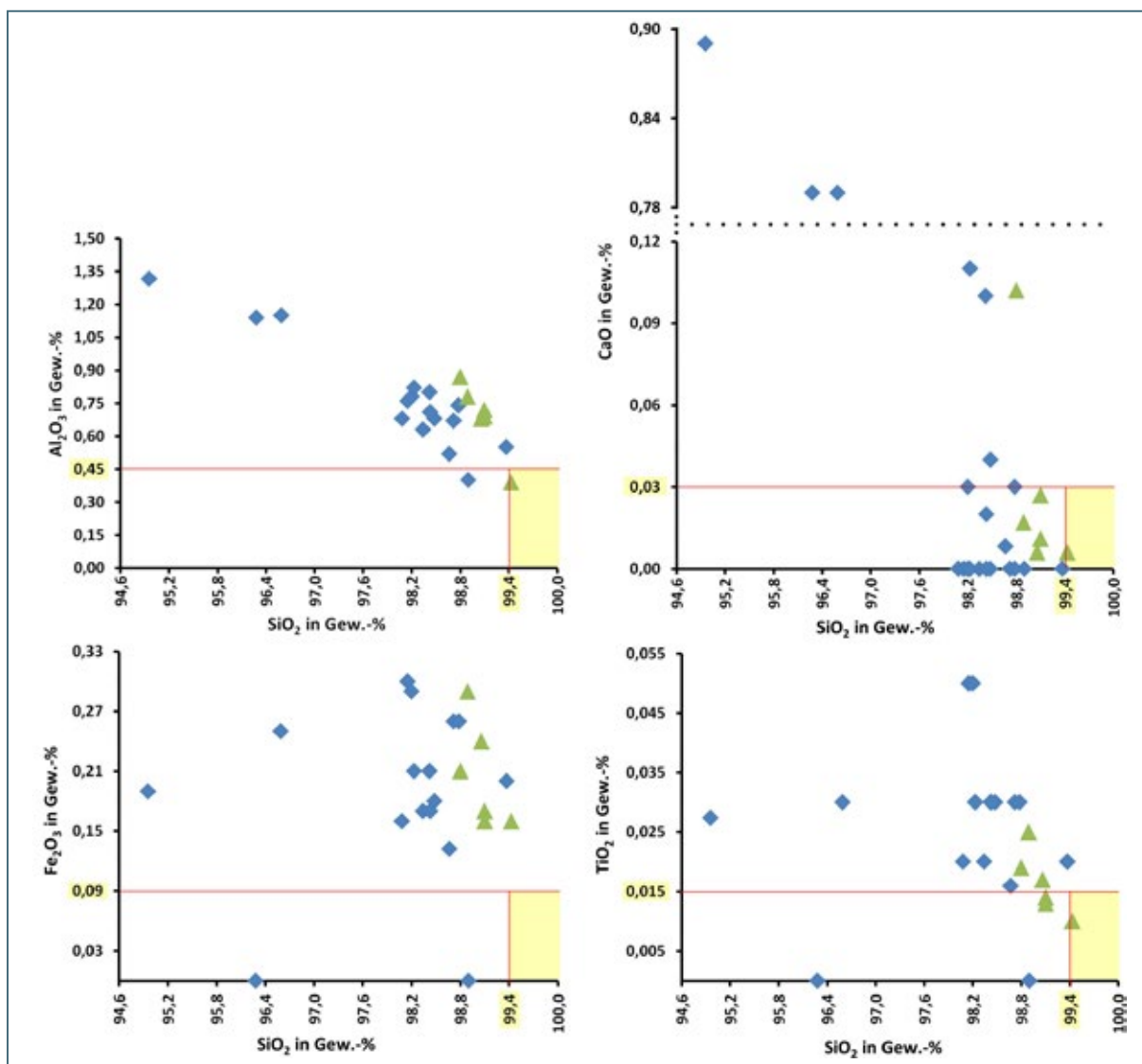
Abb. 7-13: Zusammenfassende Darstellung der chemischen Untersuchungsergebnisse aller Vollanalysen (blaue Rauten) und halbquantitativen Analysen (grüne Dreiecke) im Erkundungsgebiet 2.
