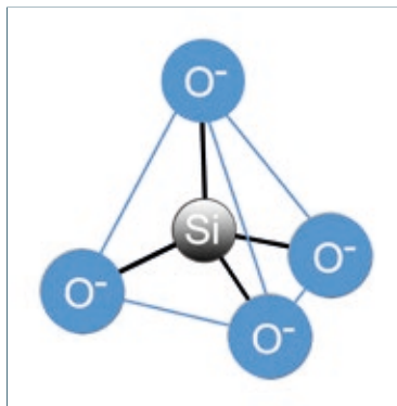
Abb. 2-1: Struktur eines \text{SiO}_4 -Tetraeders. Die Bindungen zwischen Sauerstoff und Silizium (schwarze Striche) müssen zur Herstellung von metallischem Silizium „geknackt“ werden.
