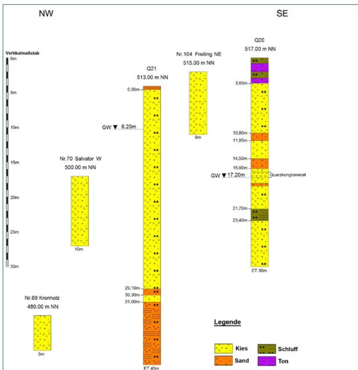
Abb. 7-22: Profilschnitt im Bereich des Forst Steinkart, nördlich Bad Griesbach (Erkundungsgebiet 4). Kieshorizonte mit Meterangabe unter Ansatzpunkt; mNN = Meter über Normal Null, ET = Endteufe, GW = Grundwasserstand)
