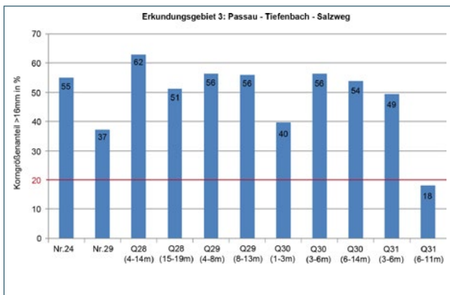
Abb. 7-19: Gewichtsprozent der Kornanteile > 16 mm. Rote Linie: Rentabilitätsgrenze (20 %).
