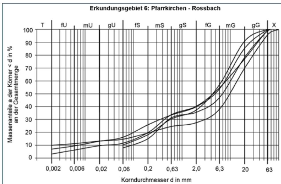
Abb. 7-39: Kornverteilung der untersuchten Kiese der Bohrung Q 33 und aus den Kiesgruben Nr. 78 Eklhub und Nr. 83 Sandberg im Erkundungsgebiet 6.
