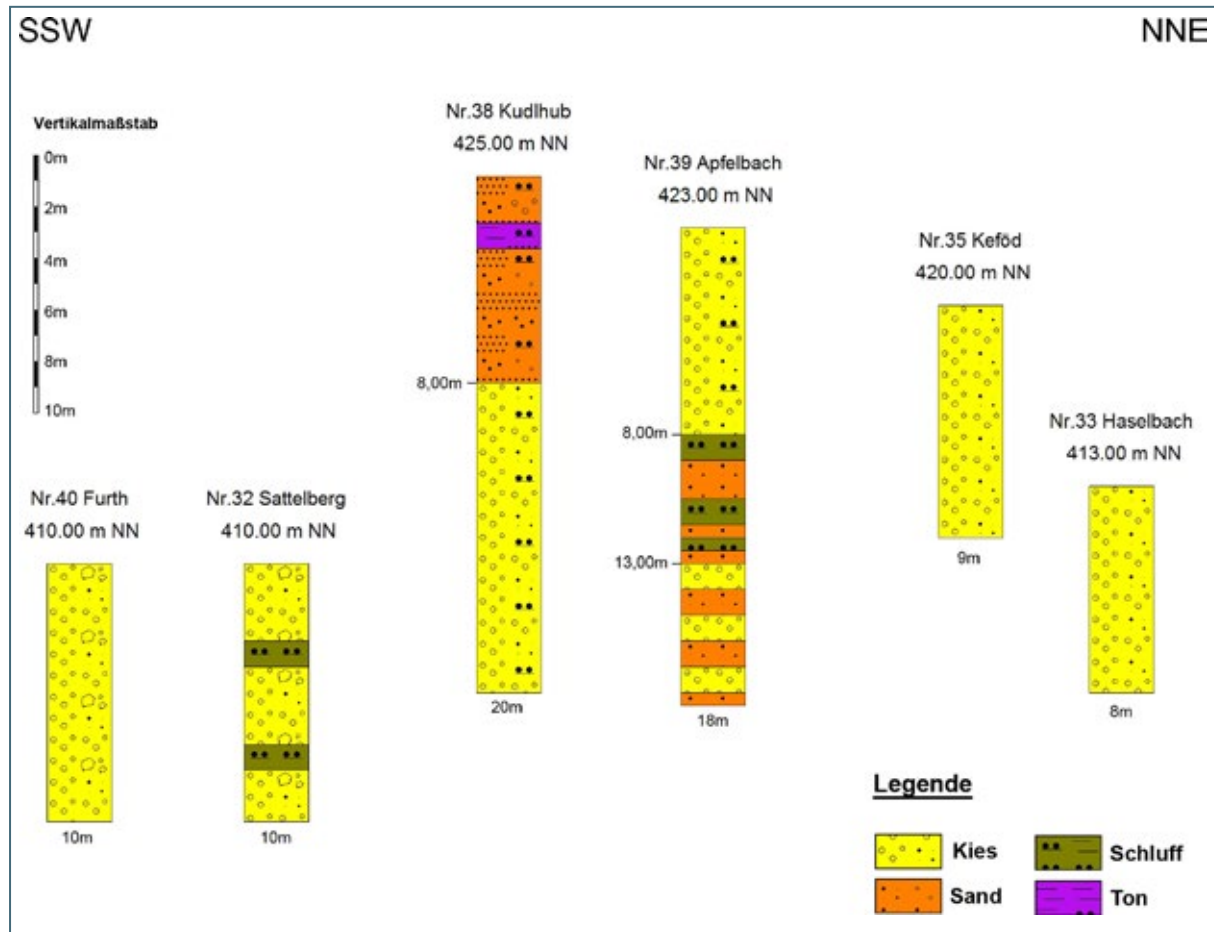
Abb. 7-36: Profilschnitt durch mehrere Kies- und Sandgruben westlich Johanniskirchen im Erkundungsgebiet 6. mNN = Meter über Normal Null
