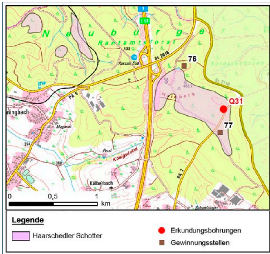
Abb. 7-16: Lage der Erkundungsbohrung Q31 und Aufschlüsse Nr. 76 und Nr. 77 südlich der Donau.
