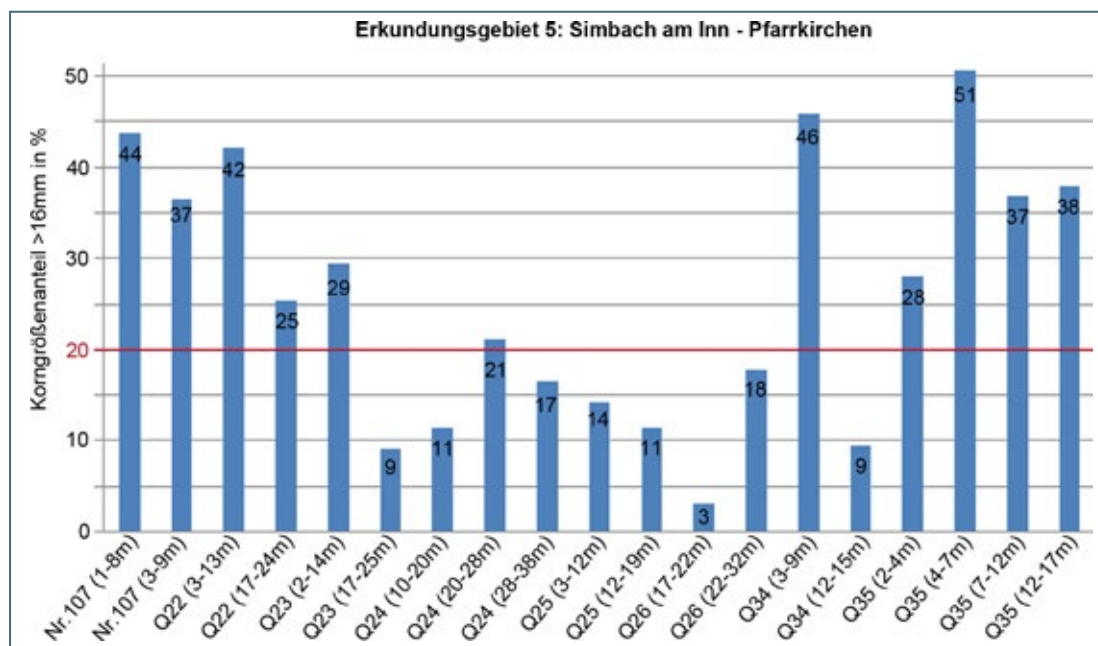
Abb. 7-33: Gewichtsprozent der Kornanteile > 16 mm. Rote Linie: Rentabilitätsgrenze (20 %)
