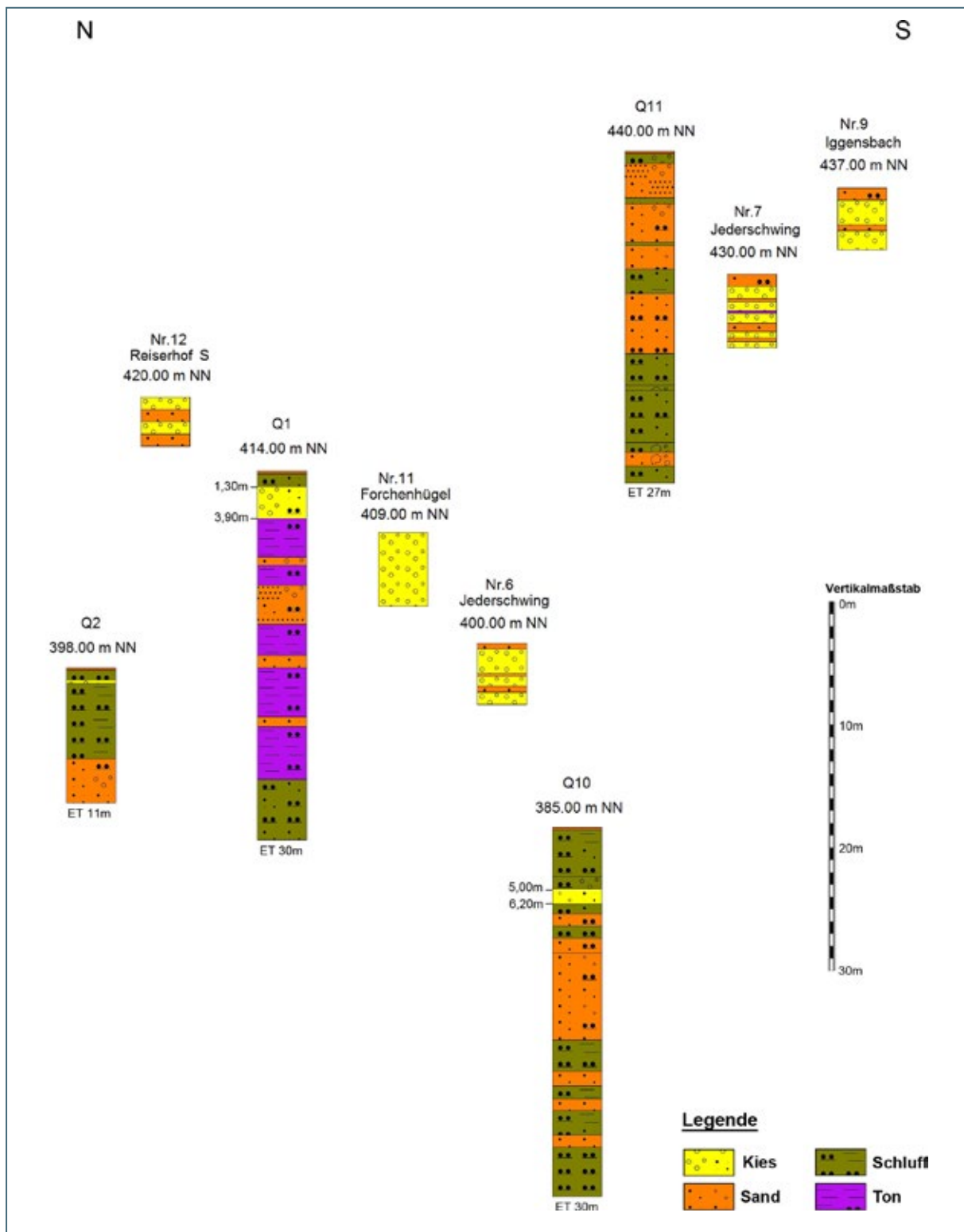
Abb. 7-3: Profilschnitt im Bereich Außernzell
