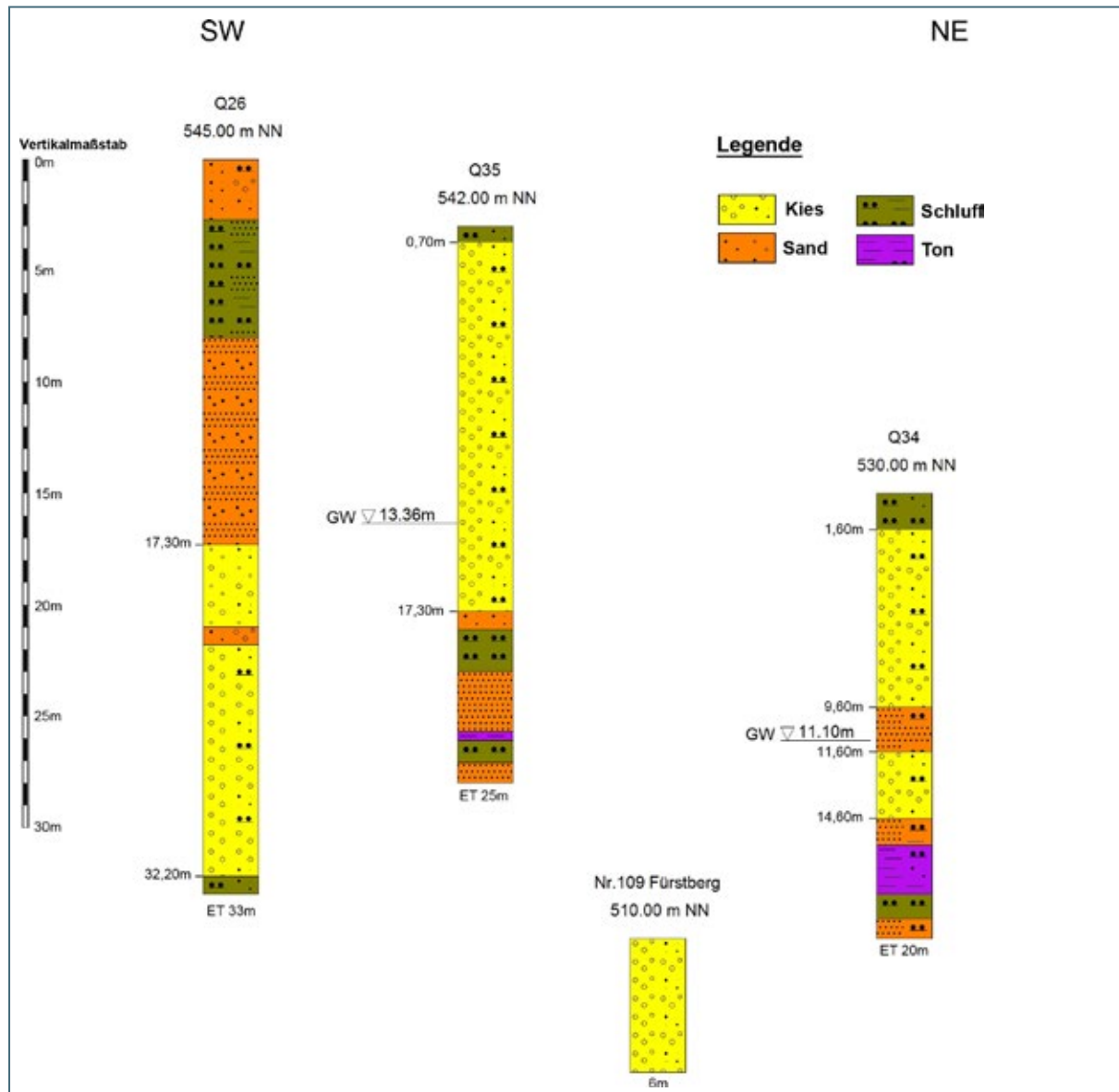
Abb. 7-30: Profilschnitt durch die Bohrungen und eine Gewinnungsstelle im Umfeld des Ortes Schellenberg, im südlichen Bereich des Erkundungsgebietes 5. Kieshorizonte mit Meterangabe unter Ansatzpunkt; mNN = Meter über Normal Null, ET = Endteufe, GW = Grundwasserstand
