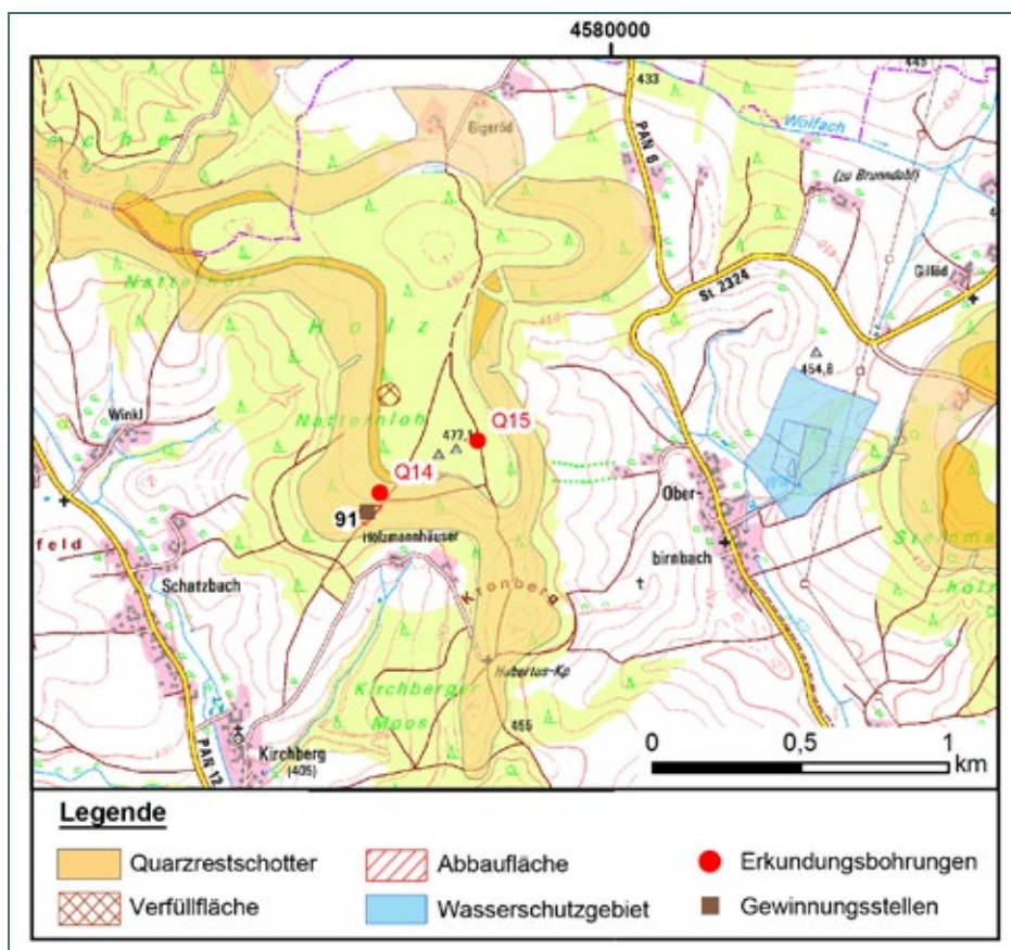
Abb. 7-24: Lage der Erkundungsbohrungen Q 14 und Q 15 und Aufschluss Nr. 91 südöstlich Egglham.
