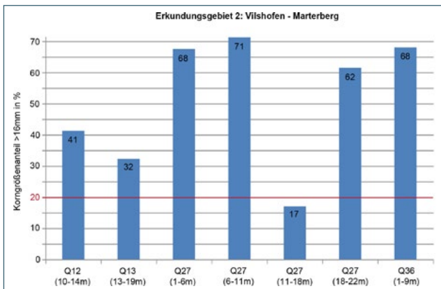
Abb. 7-12: Gewichtsprozent der Kornanteile > 16 mm. Rote Linie: Rentabilitätsgrenze (20 %)
