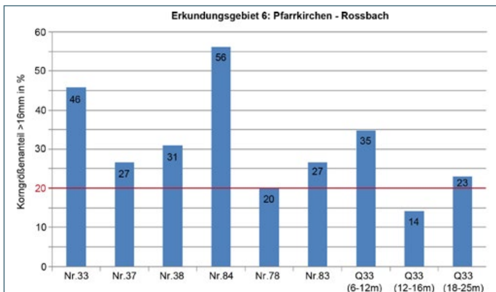
Abb. 7-40: Gewichtsprozent der Kornanteile > 16 mm. Rote Linie: Rentabilitätsgrenze (20 %)
