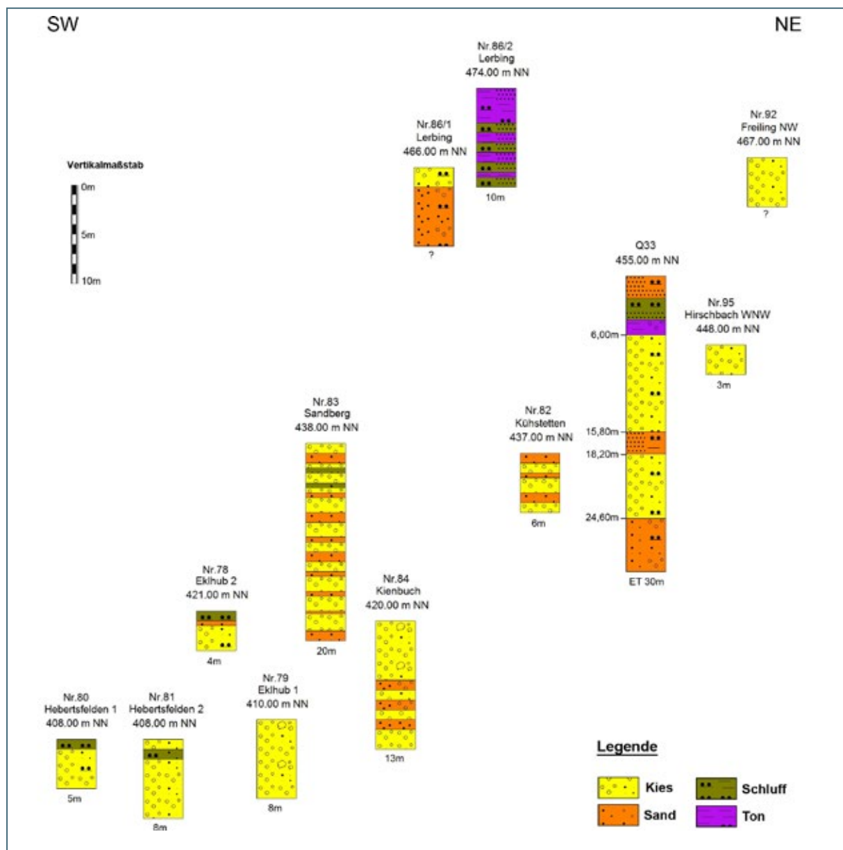
Abb. 7-38: Profilschnitt durch mehrere Kies- und Sandgruben sowie der Bohrung Q 33 südwestlich bis nordöstlich Pfarrkirchen. mNN = Meter über Normal Null, ET = Endteufe
