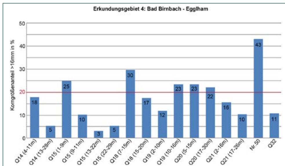
Abb. 7-27: Gewichtsprozent der Kornanteile > 16 mm. Rote Linie: Rentabilitätsgrenze (20 %).
