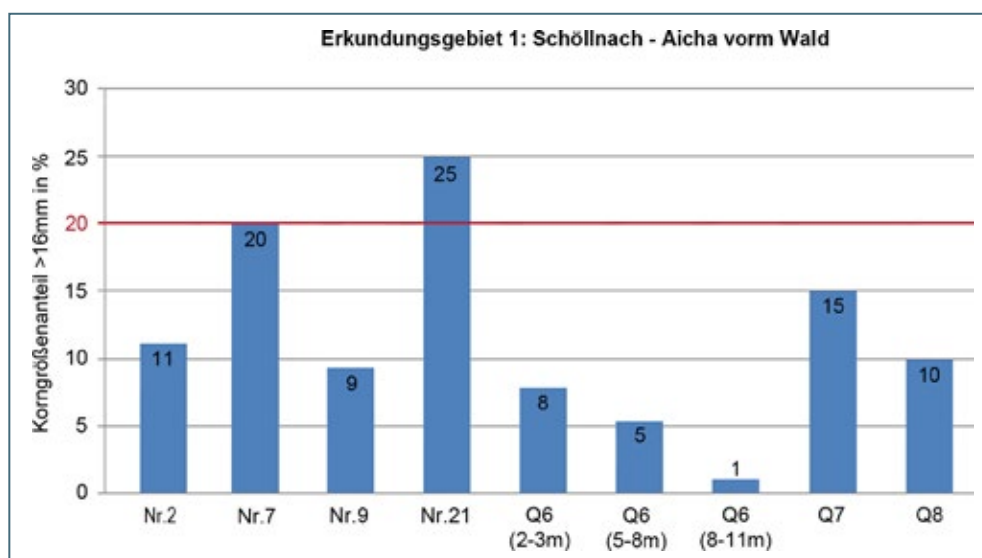
Abb. 7-6: Gewichtsprozent der Kornanteile > 16 mm. Rote Linie: Rentabilitätsgrenze (20 %)
