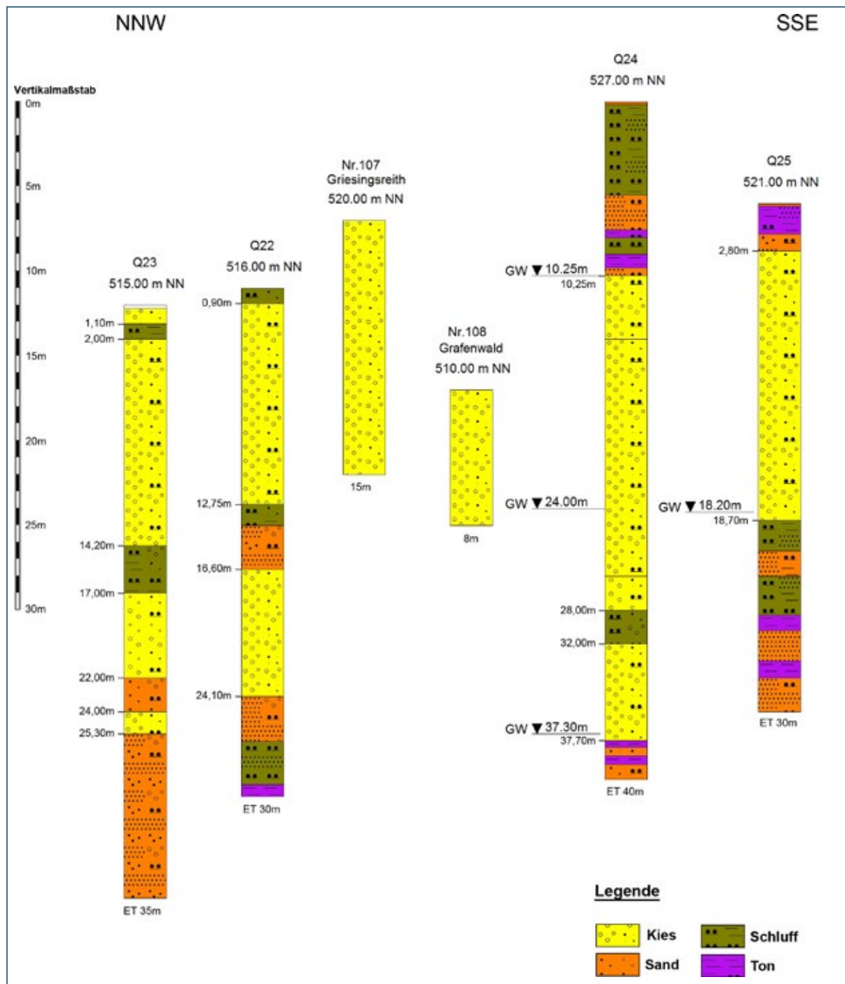
Abb. 7-31: Profilschnitt durch Bohrungen und Gewinnungsstellen im Umfeld des Ortes Kößlarn, im östlichen bis nordöstlichen Bereich des Erkundungsgebietes 5. Kieshorizonte mit Meterangabe unter Ansatzpunkt; mNN = Meter über Normal Null, ET = Endteufe, GW = Grundwasserstand
