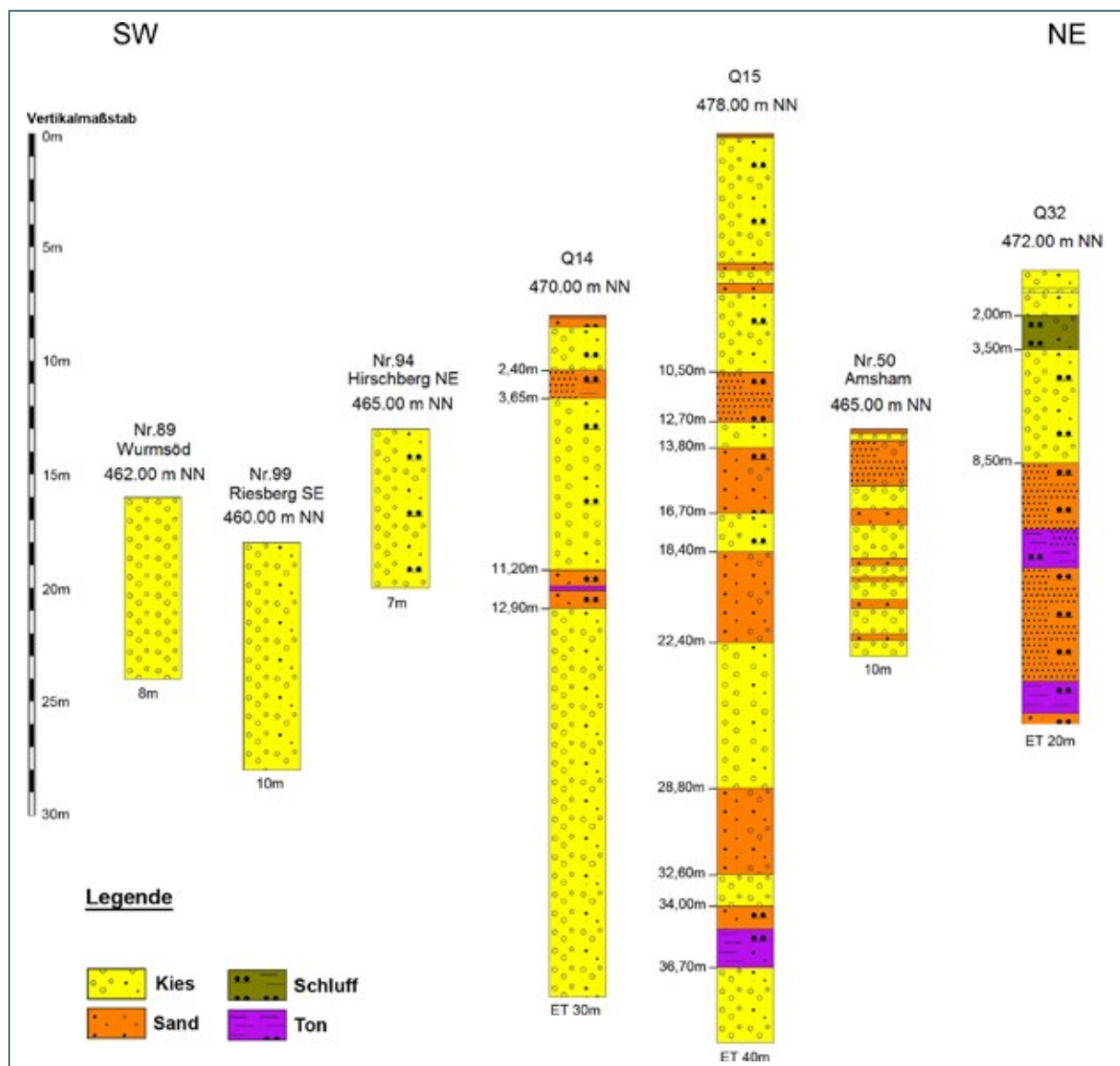
Abb. 7-25: Profilschnitt durch die Bohrungen und einige Gewinnungsstellen südlich bis südöstlich Eggldham im Erkundungsgebiet 4. Kieshorizonte mit Meterangabe unter Ansatzpunkt; mNN = Meter über Normal Null, ET = Endteufe
