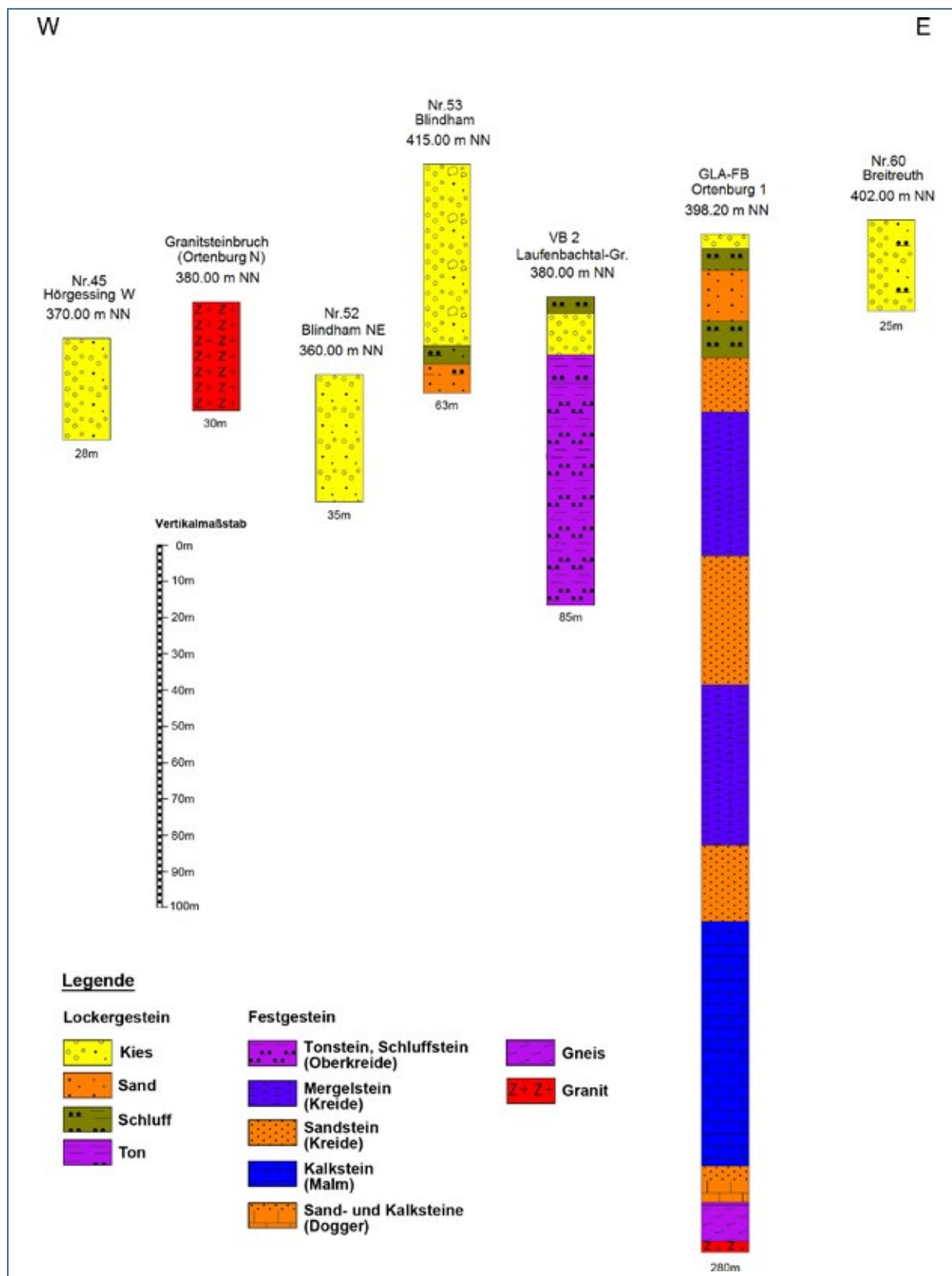
Abb. 7-44: Profilschnitt westlich bis östlich Ortenburg durch das N-S verlaufende Wolfachtal mit vier Gewinnungsstellen, zwei älteren Forschungsbohrungen und dem Ortenburger Granitsteinbruch im Erkundungsgebiet 7. mNN = Meter über Normal Null, ET = Endteufe
