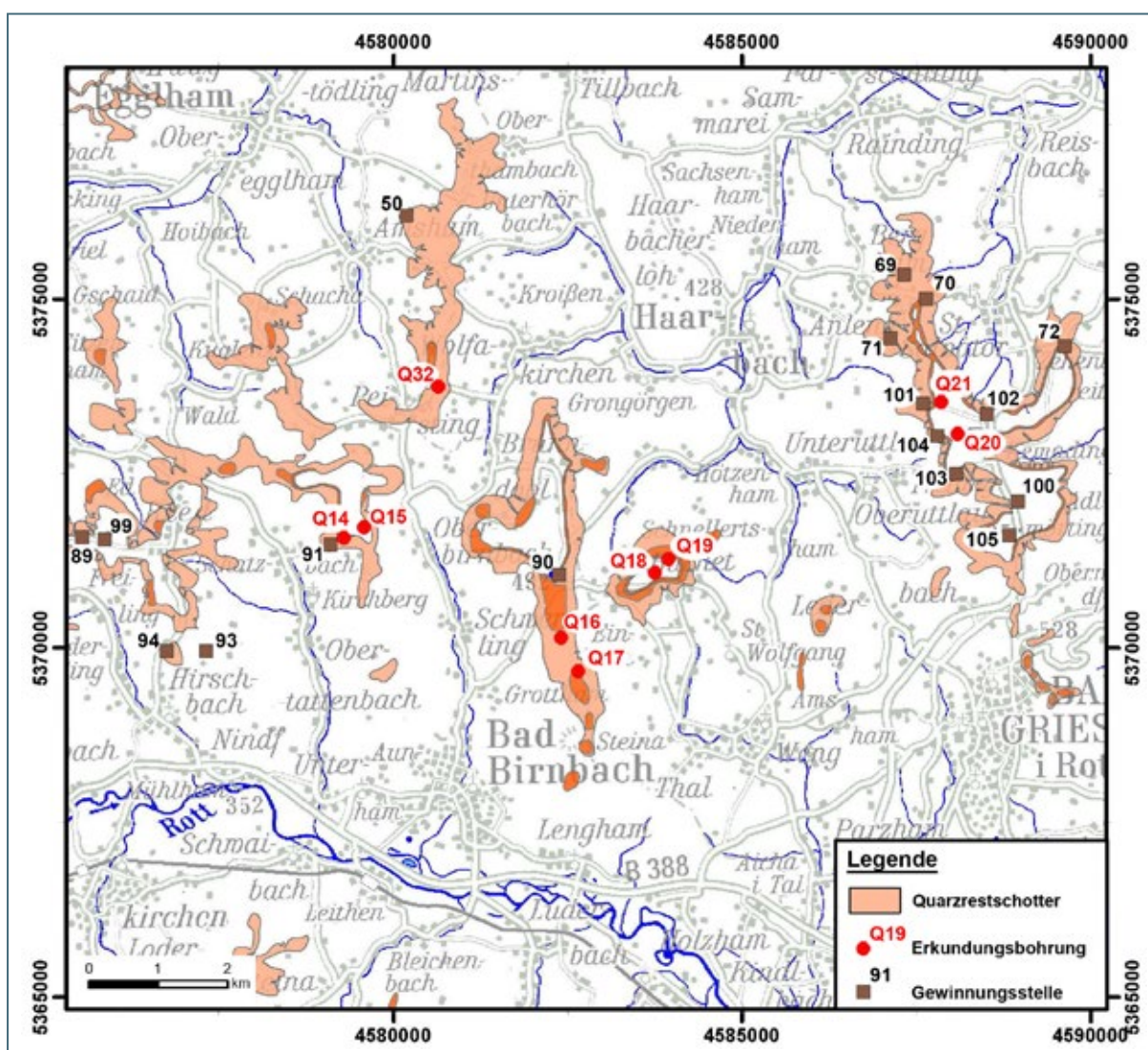
Abb. 7-21: Erkundungsgebiet 4: Bad Birnbach – Egglham
