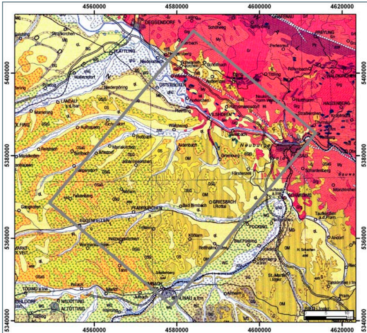
Abb. 4-2: Geologische Karte von Bayern 1:500.000, 4. Auflage (BAYERISCHES GEOLOGISCHES LANDESAMT 1996 b) mit Markierung des Untersuchungsgebietes (grauer Rahmen).
