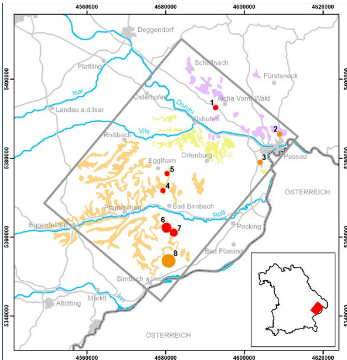
Abb. 9-1: Räumliche Übersicht der Rohstoffpotenzialflächen 1 bis 8. Rot markiert sind die Kiesvorkommen mit guter Qualität, in oranger Farbe markiert sind die Vorkommen mit ausreichender Qualität.
