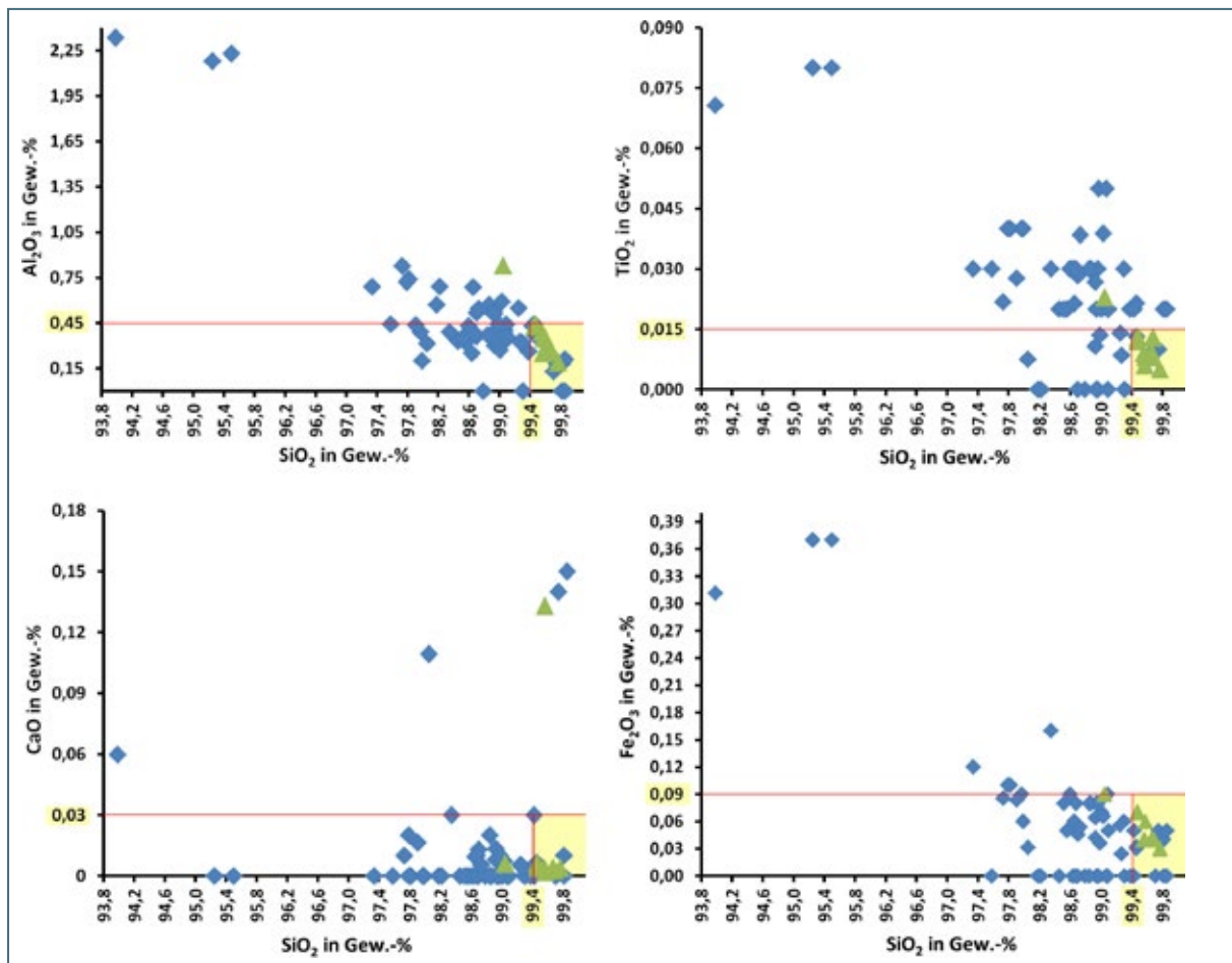
Abb. 7-34: Zusammenfassende Darstellung der chemischen Untersuchungsergebnisse aller Vollanalysen (blaue Rauten) und halbquantitativen Analysen (grüne Dreiecke) im Erkundungsgebiet 5.
