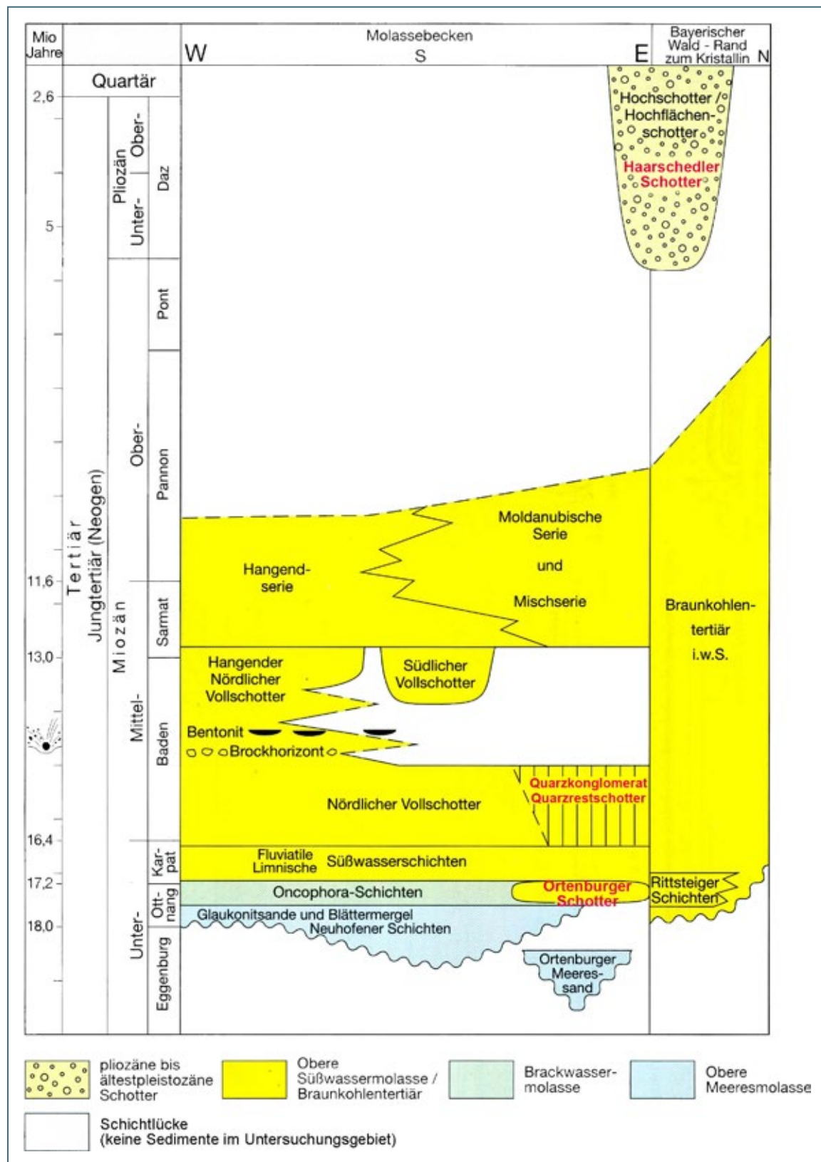
Abb. 4-3: Stratigraphische Gliederung des Tertiärs in Niederbayern – verändert nach (KEIM, GLASER & LAGALLY 2004). In roter Schrift: die in vorliegender Arbeit untersuchten Kiese.
