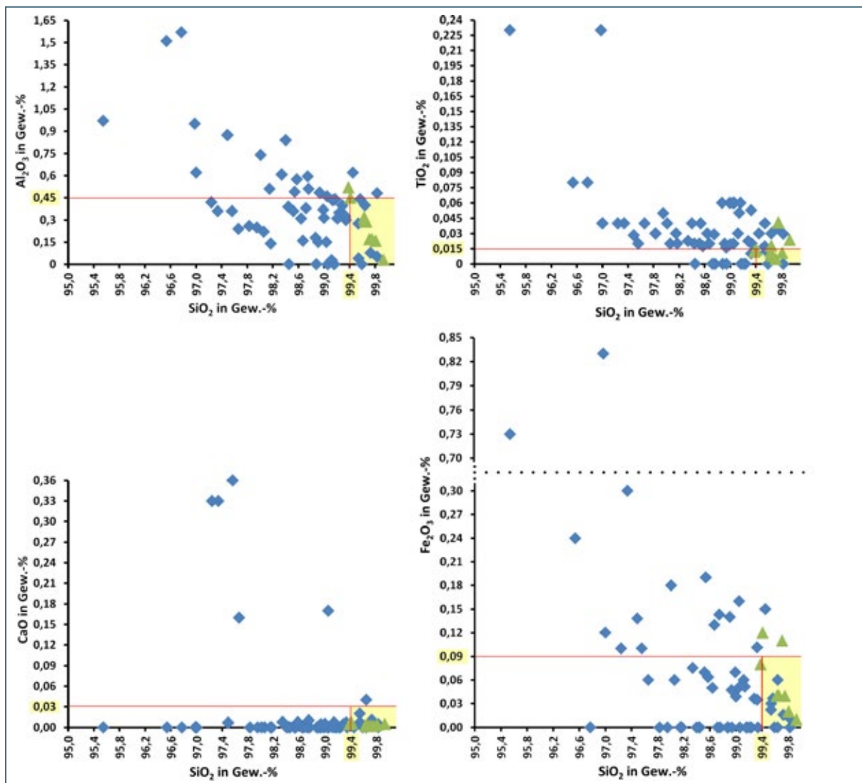
Abb. 7-28: Zusammenfassende Darstellung der chemischen Untersuchungsergebnisse aller Vollanalysen (blaue Rauten) und halbquantitativen Analysen (grüne Dreiecke) im Erkundungsgebiet 4
