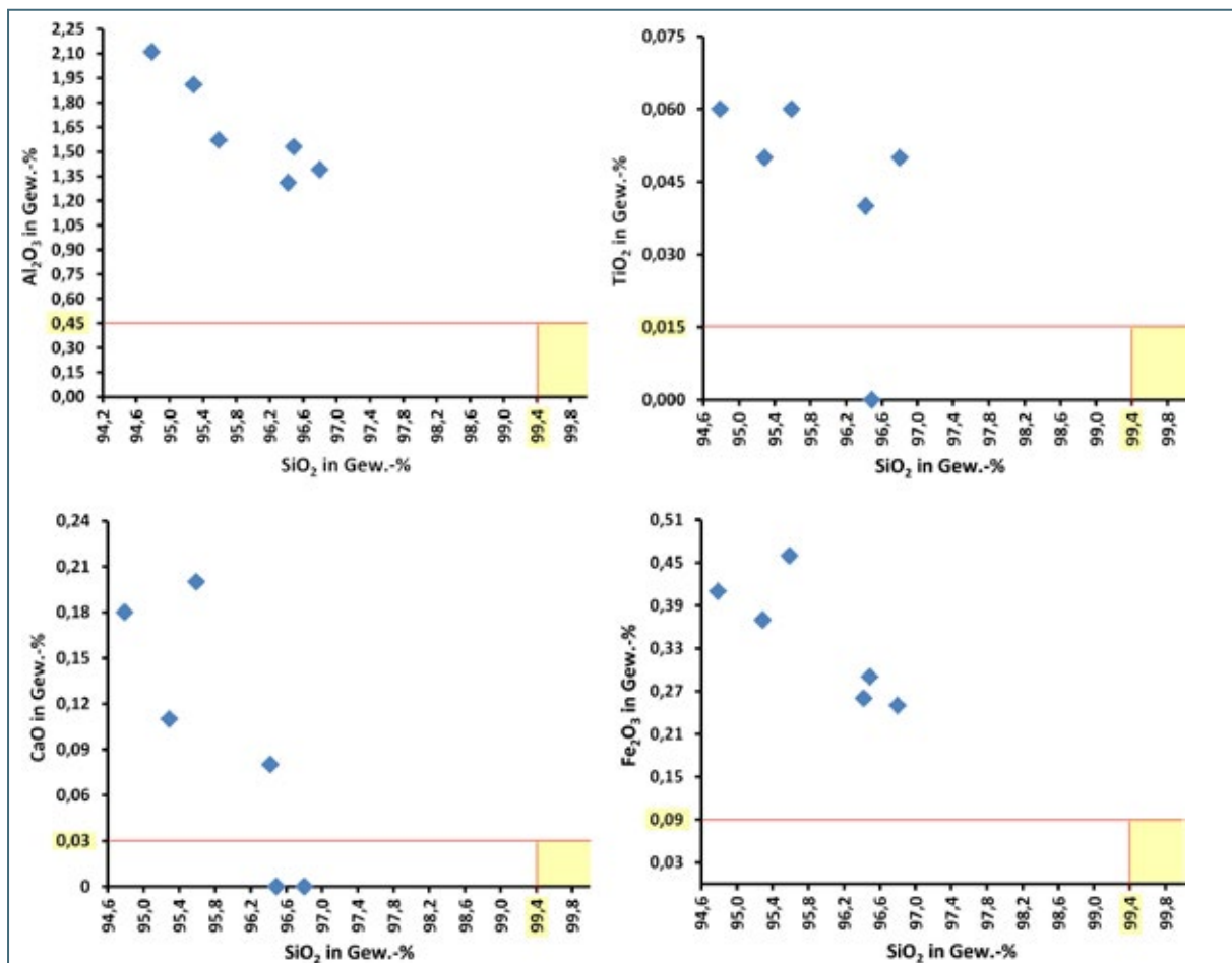
Abb. 7-48: Zusammenfassende Darstellung der Untersuchungsergebnisse aller durchgeführten Vollanalysen (blaue Rauten) des Erkundungsgebietes 7.
