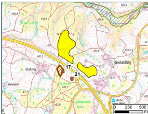
Abb. 8-1: Rohstoffpotenzialflächen Socking Nordost und Socking Ost
