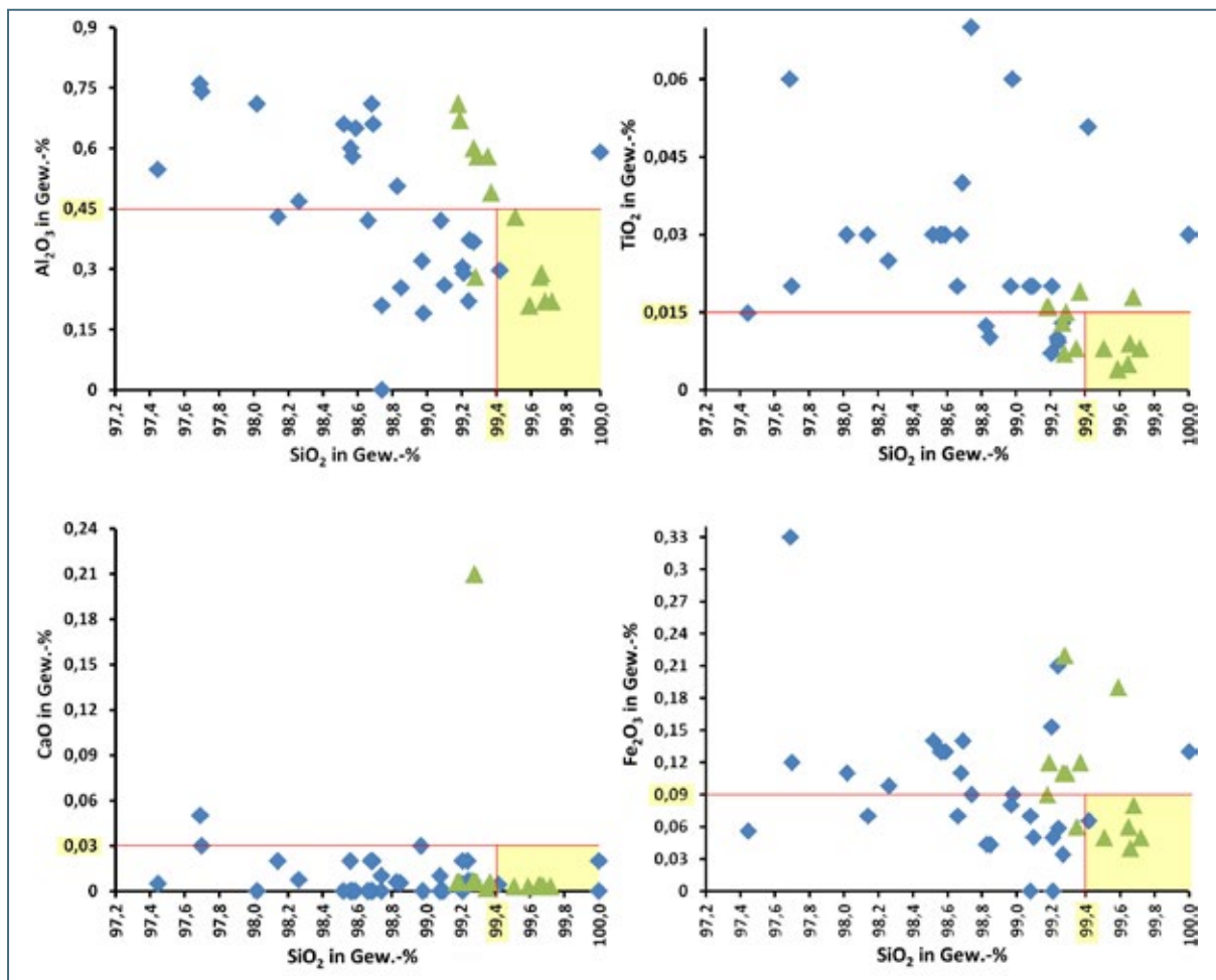
Abb. 7-20: Zusammenfassende Darstellung der chemischen Untersuchungsergebnisse aller Vollanalysen (blaue Rauten) und halbquantitativen Analysen (grüne Dreiecke) im Erkundungsgebiet 3
