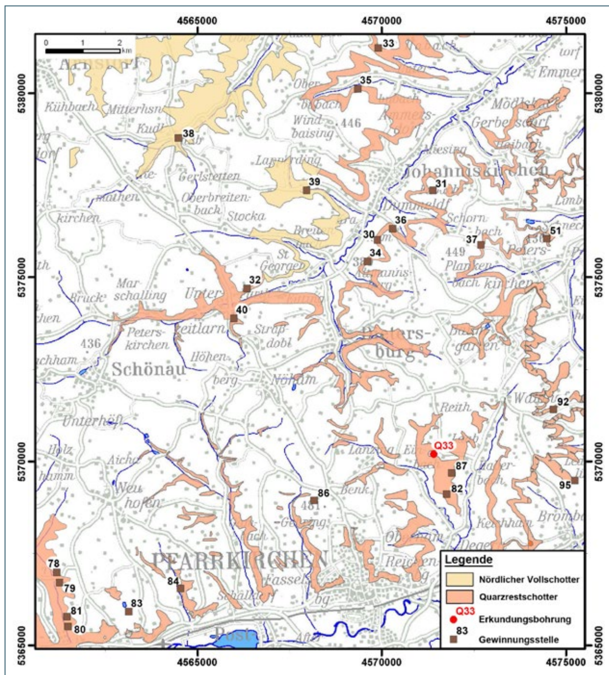
Abb. 7-35: Erkundungsgebiet 6: Pfarrkirchen – Roßbach
