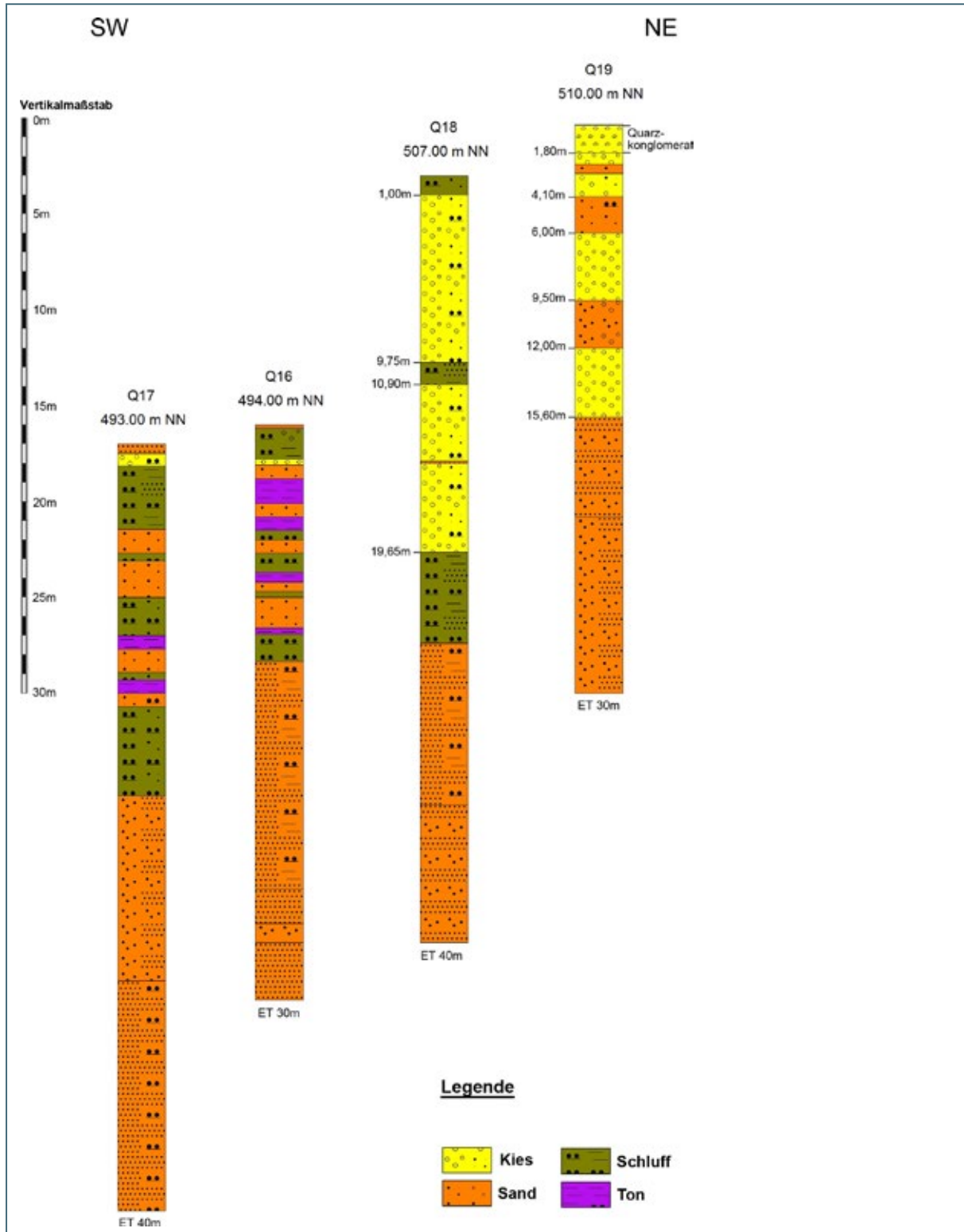
Abb. 7-23: Profilschnitt durch die Bohrungen nördlich Bad Birnbach, im zentralen Bereich des Erkundungsgebietes 4. Kieshorizonte mit Meterangabe unter Ansatzpunkt; mNN = Meter über Normal Null, ET = Endteufe
