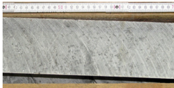
Abb. 4-14: Sulfat, massig, mit unregelmäßigen Gips-Butzen, Gips 13, Ahlstadt, 92,4 m - 92,7 m
