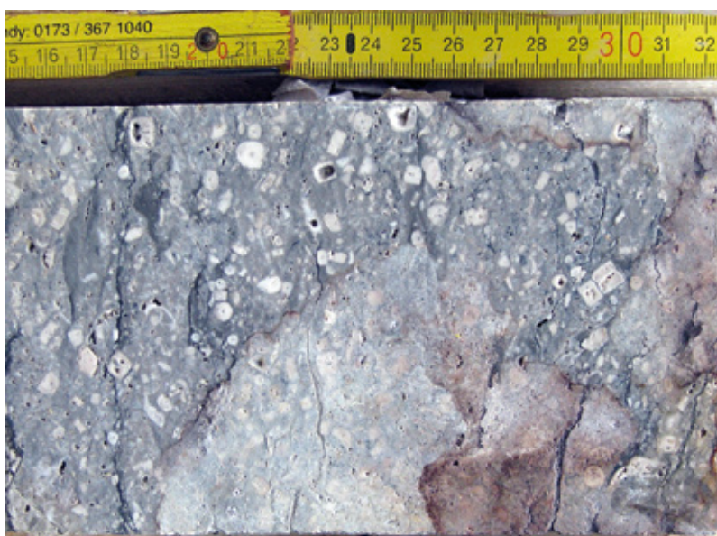
Abb. 4-3: Trochitenkalk des mo1, Bohrung Gips 8, Döberschütz, 26,1 m - 26,35 m
