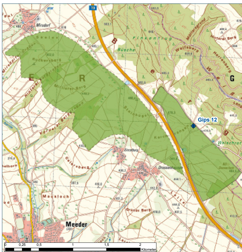
Abb. 7-1: Rohstoffpotenzialflächen nordöstlich Meeder; Untertageabbau in ca. 60 m u. GOK. Erkundete Mächtigkeit in Bohrung Gips 12: ca. 13,3 m. Integriertes Verhältnis Gips/ Anhydrit: 72/17
