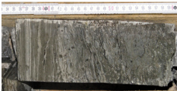
Abb. 4-13: Aufgearbeiteter Sulfat. Gips 12, Drossenhausen, 61,35 m - 61,6 m
