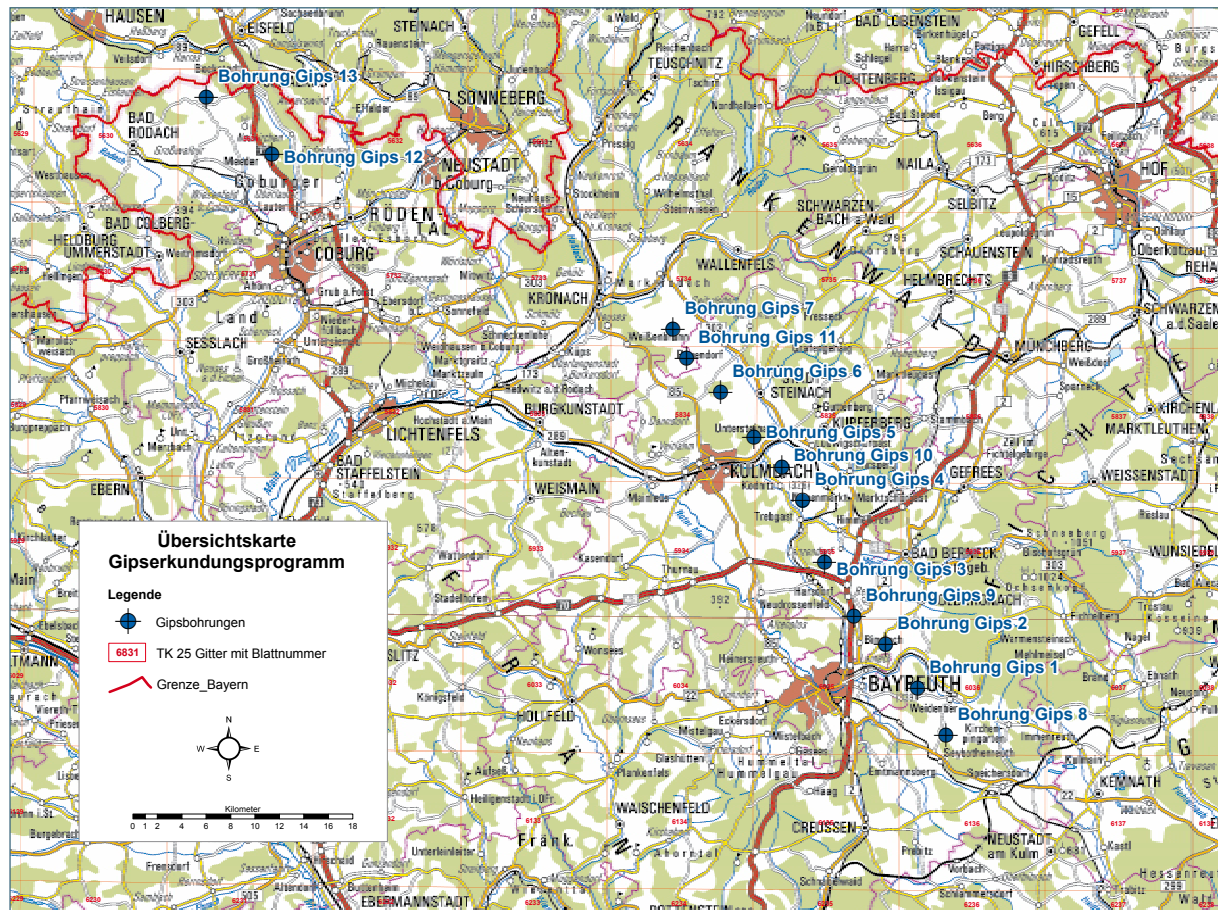
Abb. 3-1: Arbeitsgebiet mit Lagepunkten
