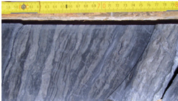
Abb. 4-11: Laminierter Sulfat. Gips 4, Hegnabrunn, 72,6 m - 72,8 m
