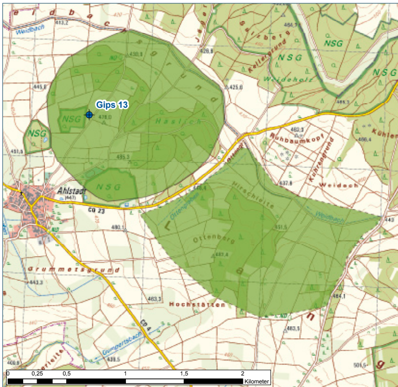
Abb. 7-2: Rohstoffpotenzialflächen nordöstlich Ahlstadt. Untertageabbau in ca. 85 m u. GOK. Erkundete Mächtigkeit in Bohrung Gips 13: ca. 13 m. Integrierte Verhältnisse Gips/Anhydrit: 78/6
