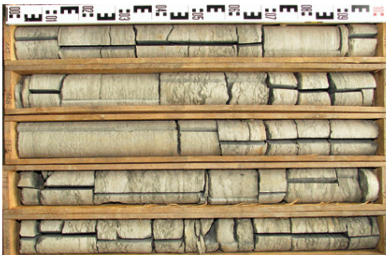
Abb. 4-7: Typischer Unterer Muschelkalk (Wellenkalk), Bohrung Gips 2, Bindlach, von links oben bis rechts unten: 115 m - 120 m
